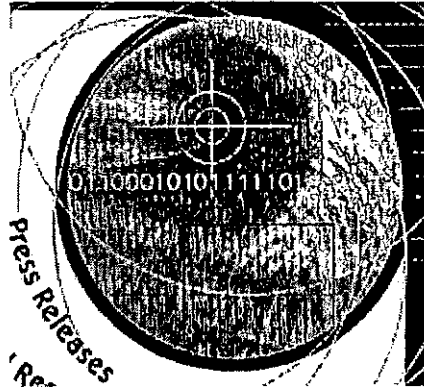
Fig. 1-6 Iris
